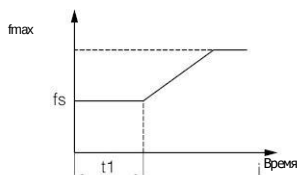
Рисунок F1-1. Начальная частота
