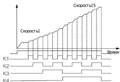
Рисунок F7-1 Многоскоростной режим работы
