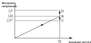
Рис. F5-4. Режим управления напряжением 0 F0----- — заданная частота; V0----- — номинальное напряжение, соответствующее заданной частоте; U*/U1* — установочное значение параметра F5.13 конкретного канала.
