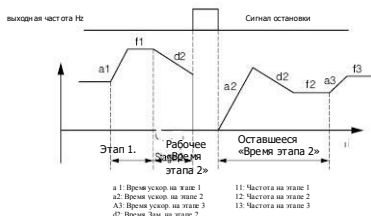
Рис. F9-5 Режим запуска ПЛК 2
