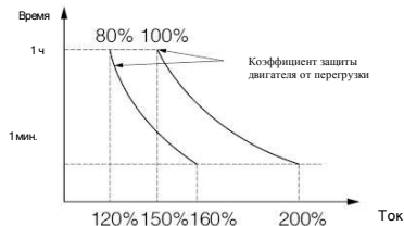
Рис. FA-2 Настройка коэффициента защиты двигателя от перегрузки Коэффициент рассчитывается по приведенной ниже формуле:
