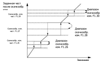
Рис. F1-6. Скачкообразно изменяемые частоты
