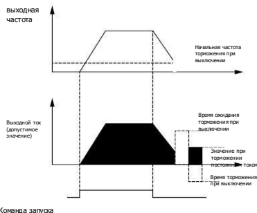
Рис. F1-4. Торможение постоянным током на этапе останова
