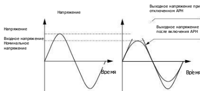
Рис. FC-2 Функция АРН
