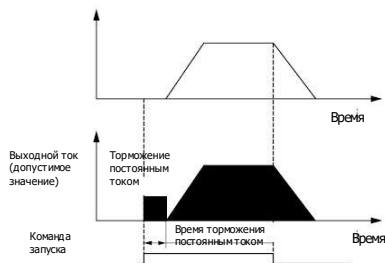
Рисунок 1-2. Торможение постоянным током на этапе запуска
