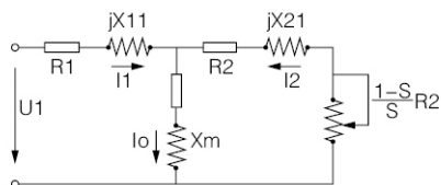
Рис. F2-1. Эквивалентная схема асинхронного двигателя для работы в установившемся режиме
