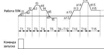
Рис.F9-2 Сохранение последнего этапа после одиночного цикла
