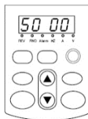
Рис. 3-2. Отображение параметров в состоянии останова (индикация заданной частоты «50.0»)
