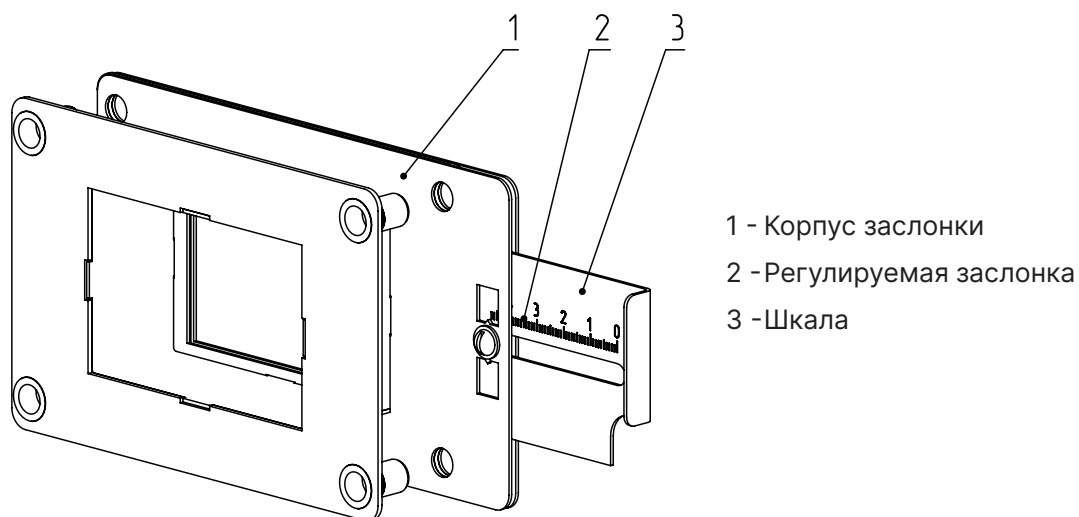
Рис.11 Заслонка вентилятора
