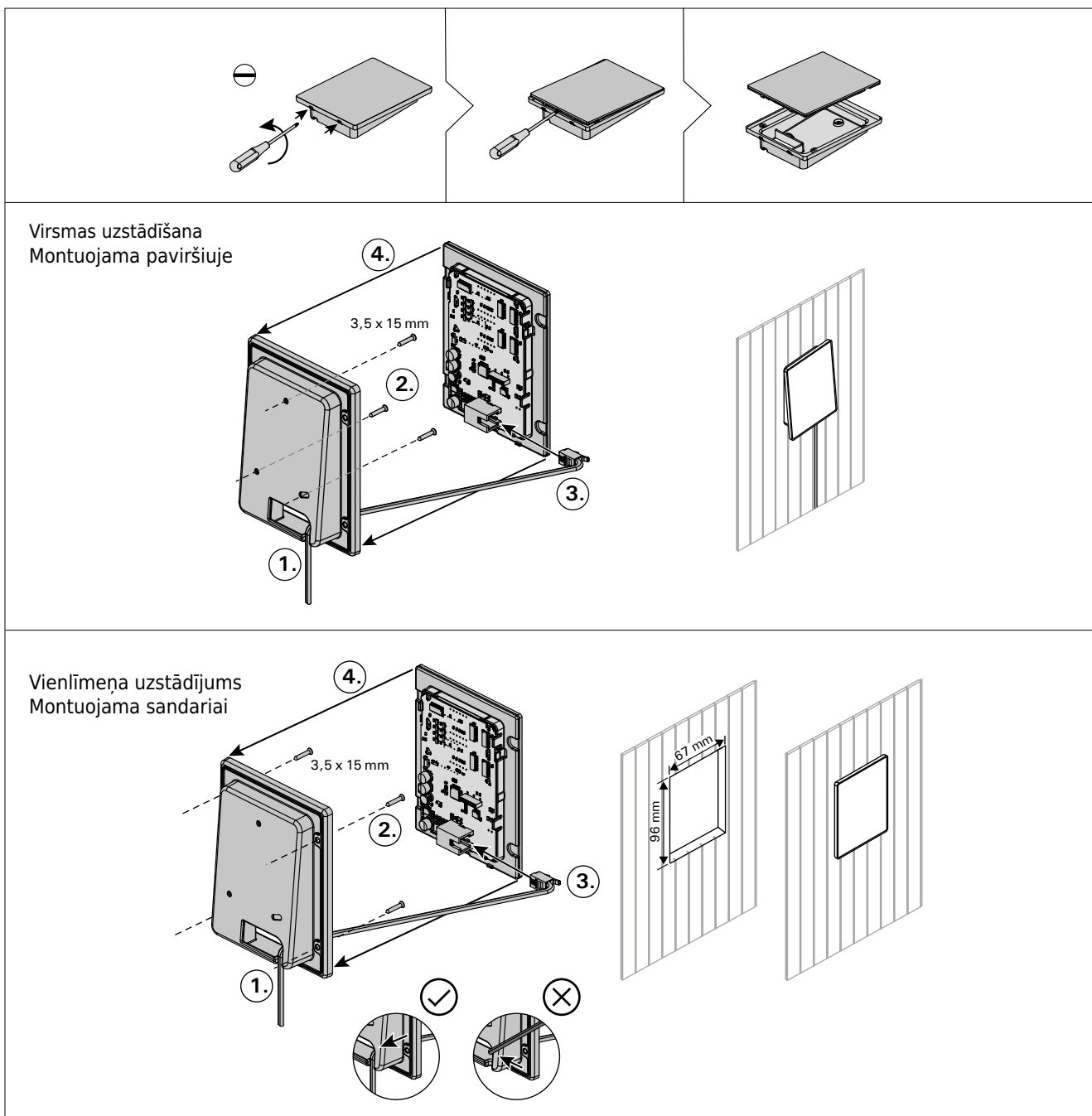
8. zīmējums. Vadības panela piestiprināšana 8 pav. Valdymo pulto instaliavimas
