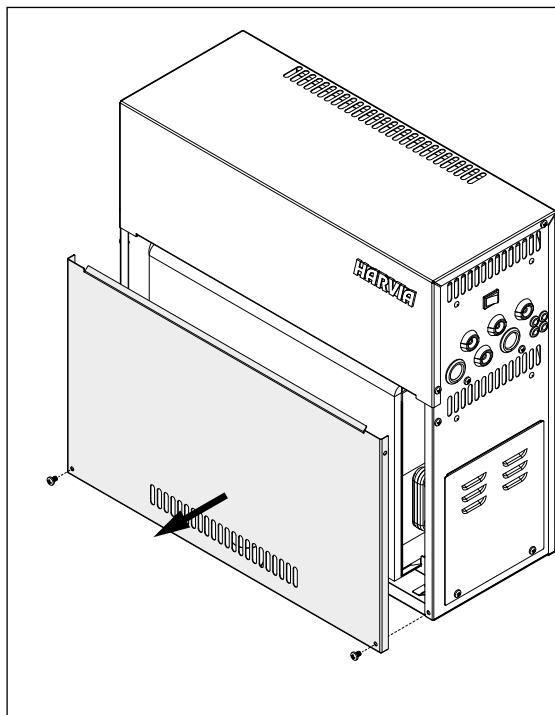
Rysunek 9. Restartowanie bezpiecznika termicznego Obrázek 9. Resetování ochrany proti přehřátí
