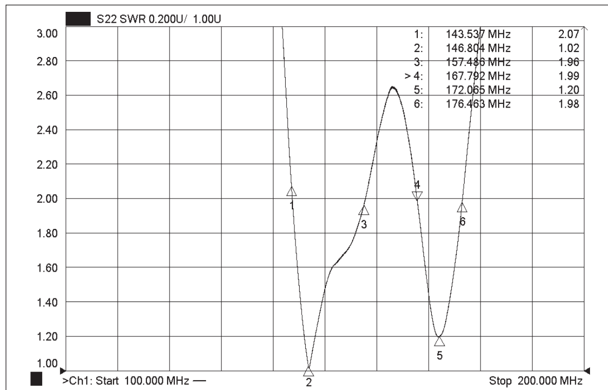
График КСВ
