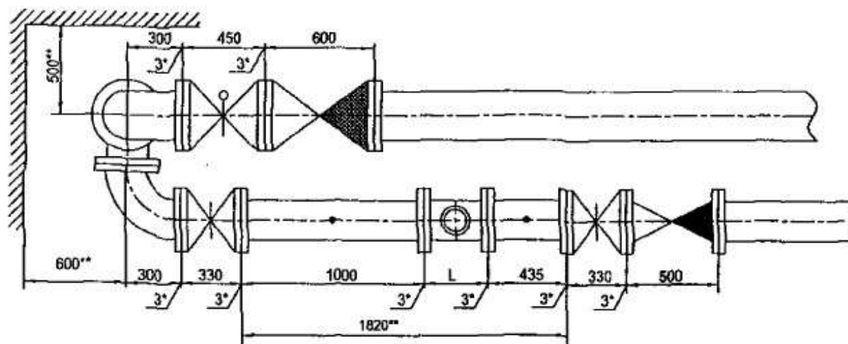
Установка счетчика dy=200 мм на хозяйственно-питьевой линии с раздельной системой хозяйственно-питьевого и противопожарного водопроводов на вводе диаметром 250 мм. Схема водомерного узла.
