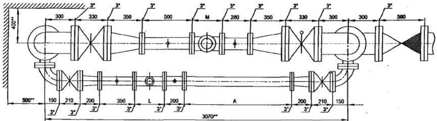
Установка счетчика d_u=65 мм на хозяйственно-питьевой линии и счетчика d_u=100 мм на пожарно-резервной линии в водомерном узле на вводе диаметром 200 мм. Схема водомерного узла.
