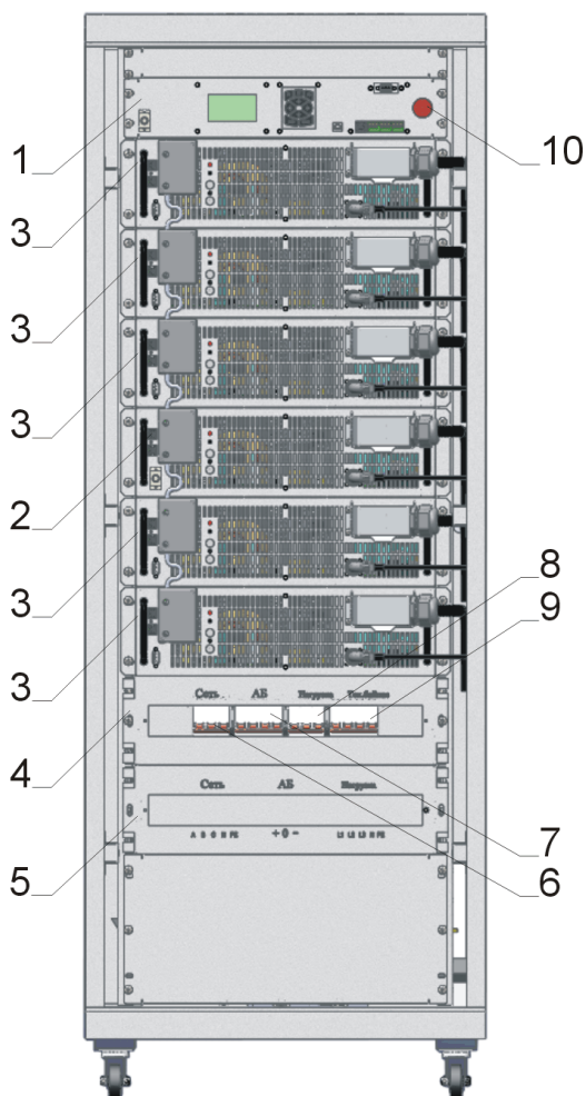
Рис. 1 ИБП ДПК-3/3-60-380. Вид спереди.
