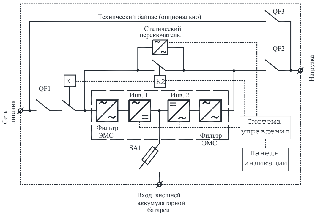
Рис. 3 Структурная схема ИБП
