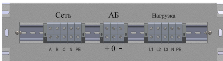
Рис.4 Клеммные колодки ИБП
