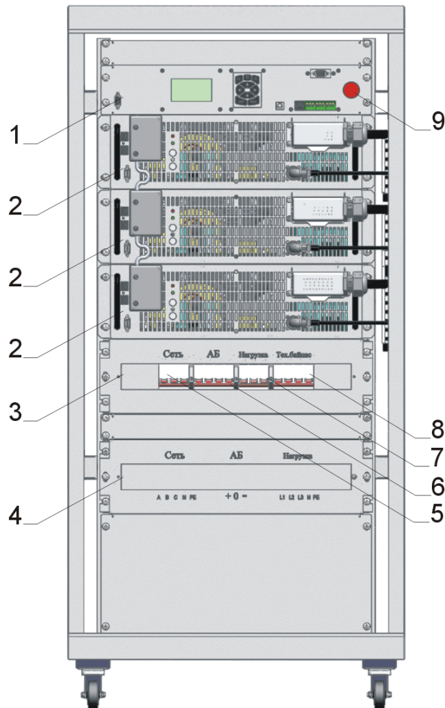
Рис. 1 ИБП ДПК-3/3-30-380. Вид спереди.
