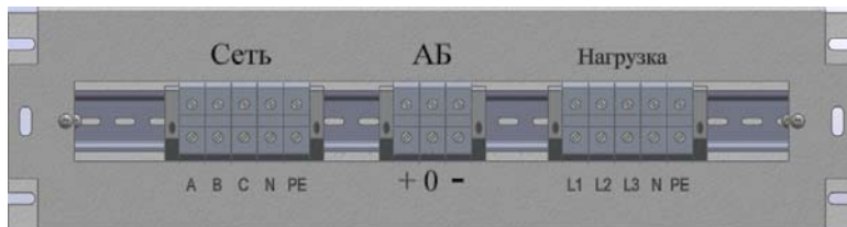
Рис.4 Клеммные колодки ИБП
