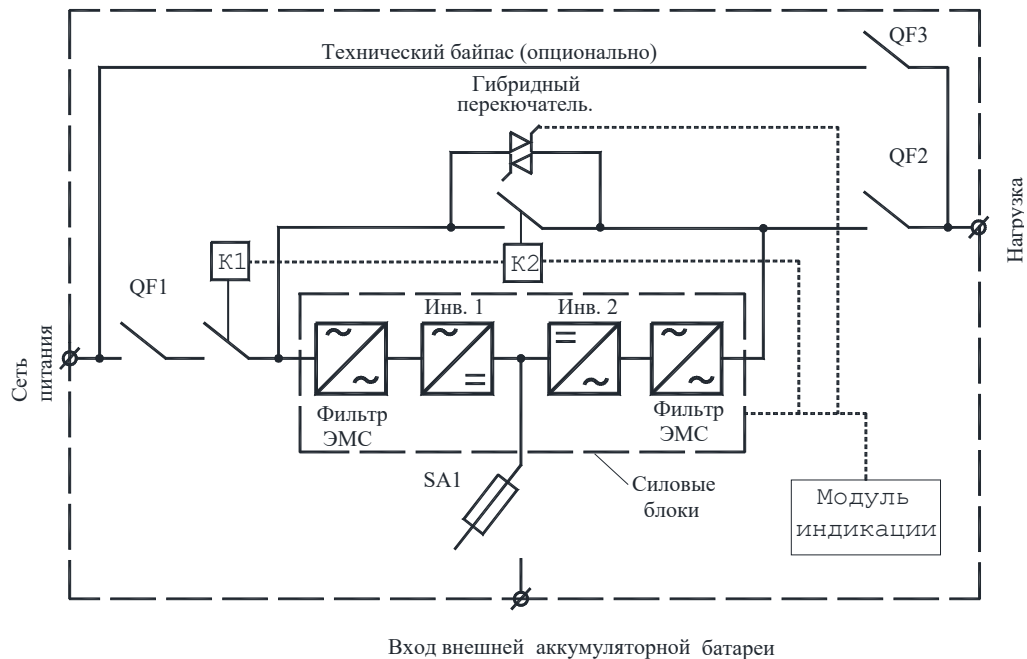
Рис. 3 Структурная схема ИБП
