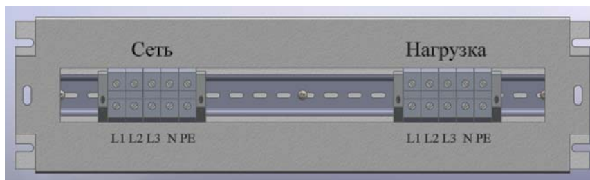
Рис.4 Клеммные колодки ИБП
