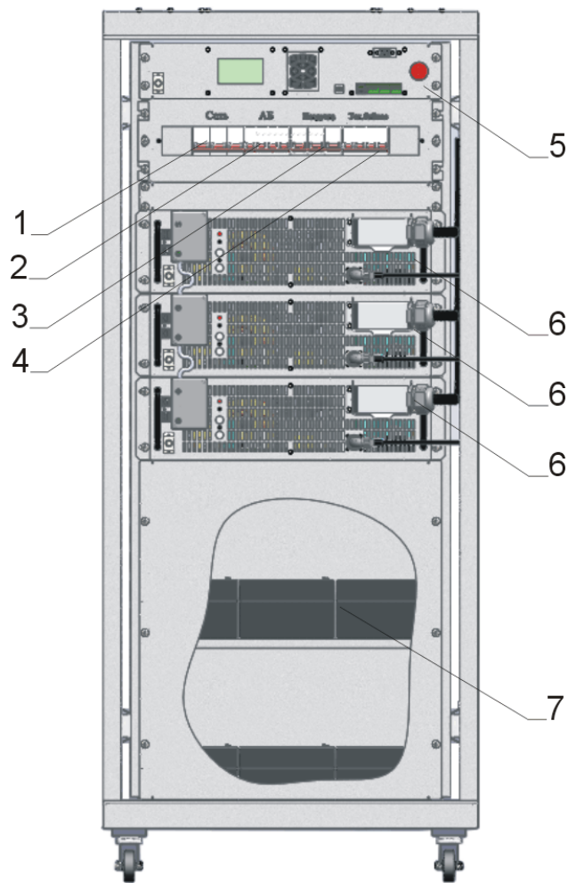
Рис. 1 ИБП ДПК-3/3-30-380. Вид спереди.
