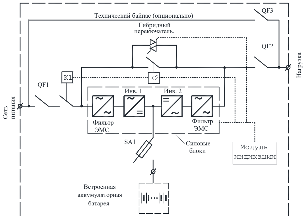
Рис. 3 Структурная схема ИБП
