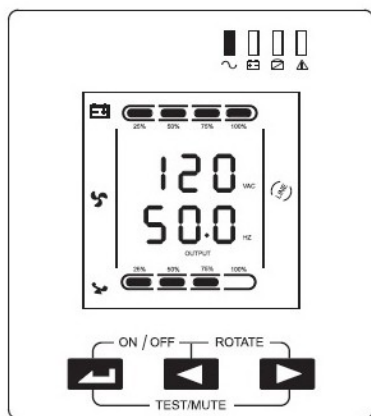
Панель управления Корпус Rack Tower
