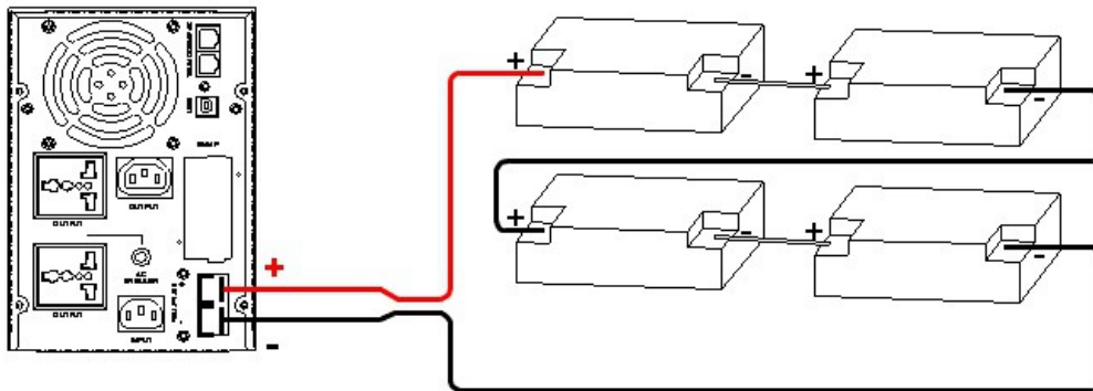
Корпус Tower. Схема подключения аккумуляторных батарей Напряжение постоянного тока U=48V .
