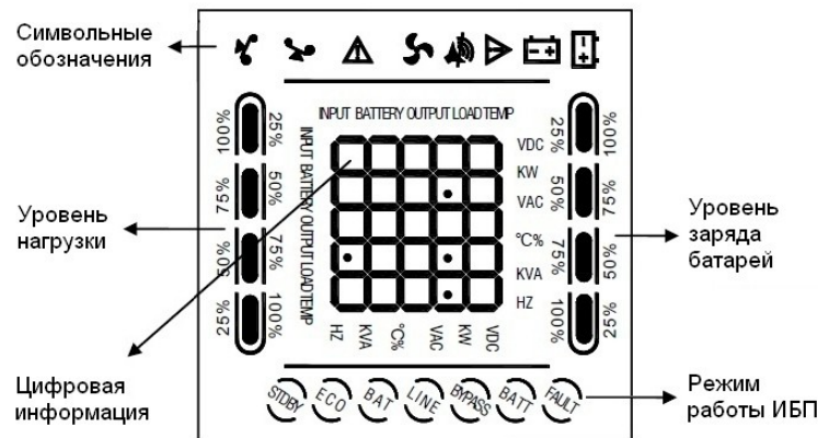
LCD-дисплей. Корпус Rack Tower.
