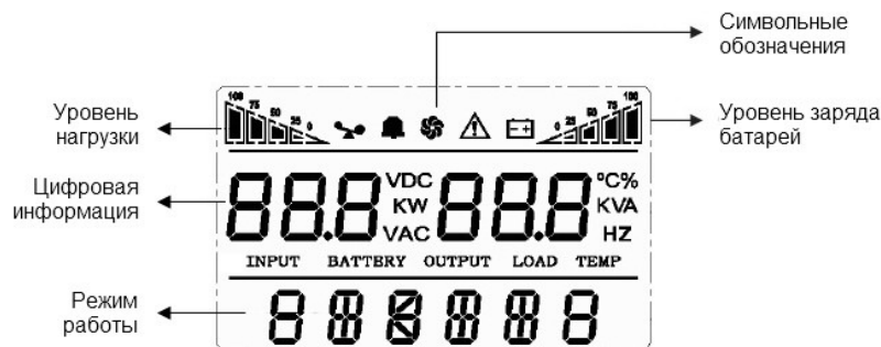
LCD-дисплей. Корпус Tower.
