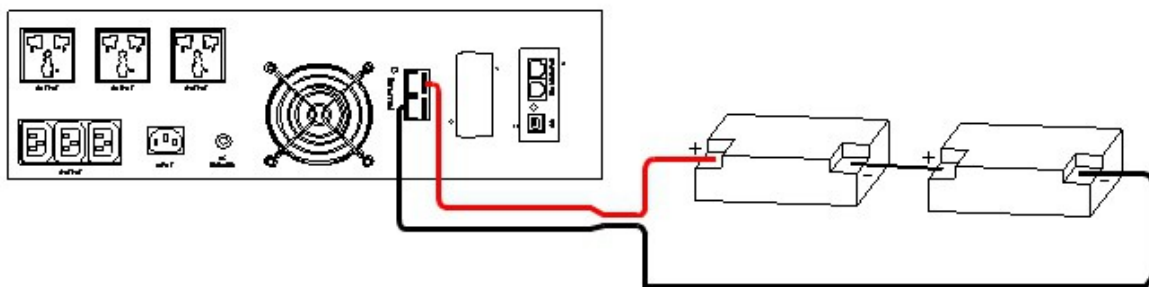
Корпус Rack Tower. Схема подключения аккумуляторных батарей Напряжение постоянного тока U=24V .
