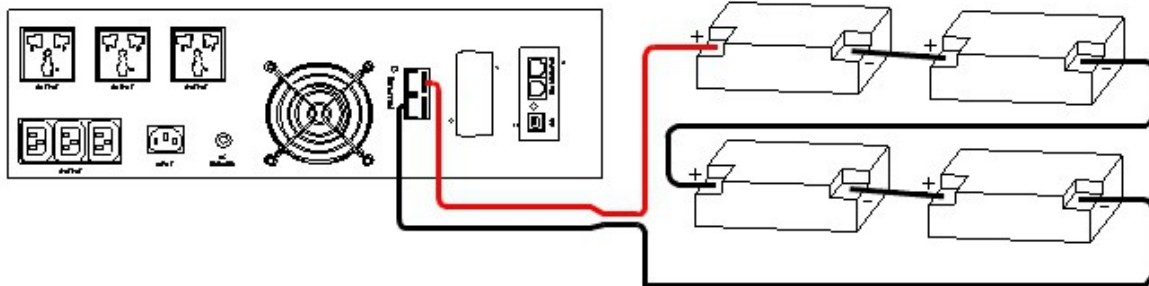
Корпус Rack Tower. Схема подключения аккумуляторных батарей Напряжение постоянного тока U=48V .
