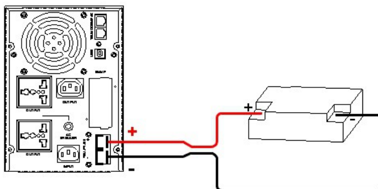
Корпус Tower. Схема подключения аккумуляторных батарей. Напряжение постоянного тока U=12В .
