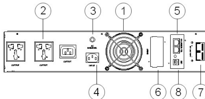
Корпус Rack Tower. Задняя панель ИБП 1 кВА
