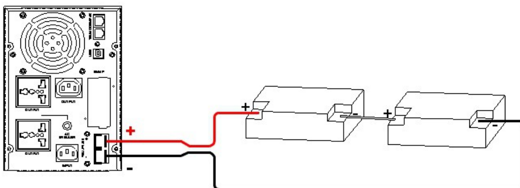
Корпус Tower. Схема подключения аккумуляторных батарей Напряжение постоянного тока U=24В .
