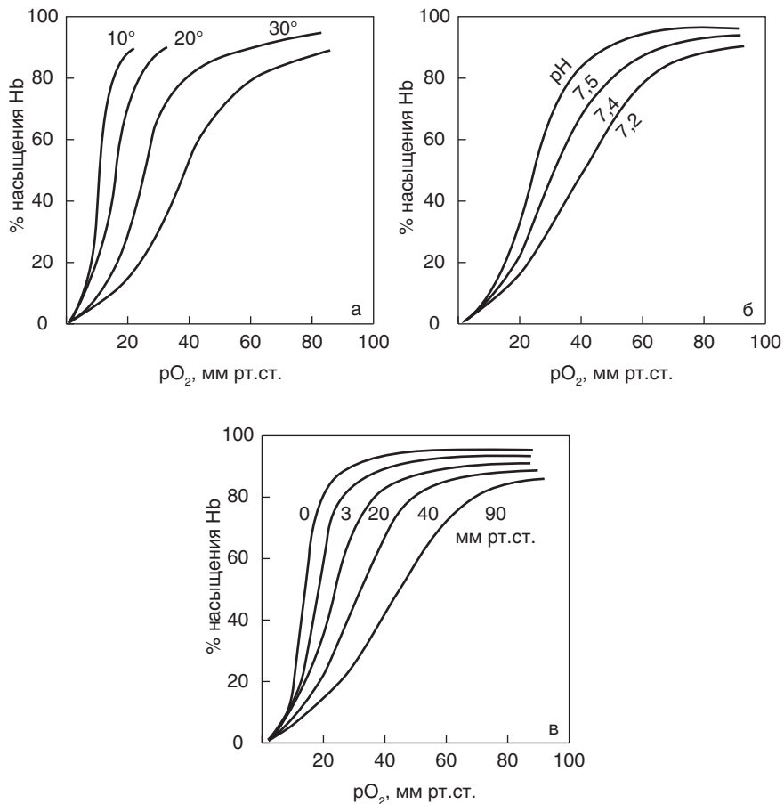
Рис. 1.4. Влияние различных факторов на кривую диссоциации оксигемоглобина: а — температуры; б — pH; в — p_aCO_2 [8]
