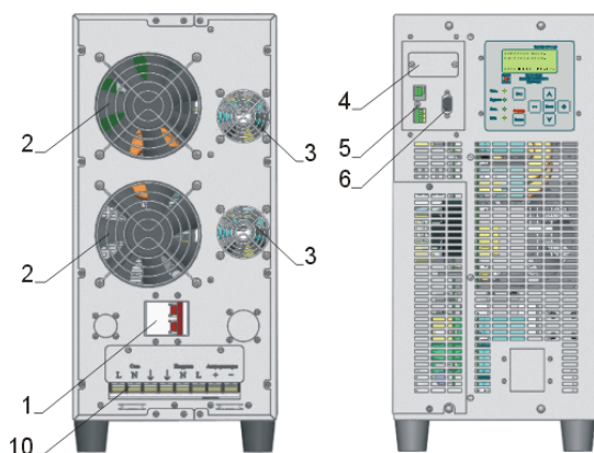
б) ДПК-1/1-6-М, ДПК-1/1-10-М
