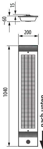
Frontansicht
