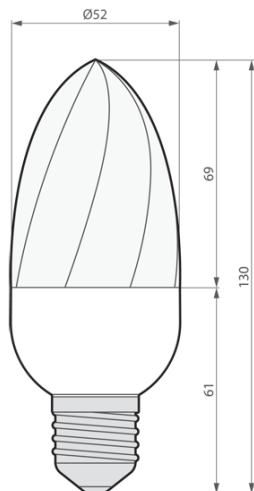
Рисунок 1 – Габаритные размеры.
