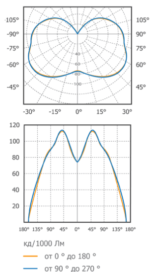
Рисунок 2 – КСС.
