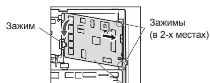
Печатная плата внешнего ввода/вывода
