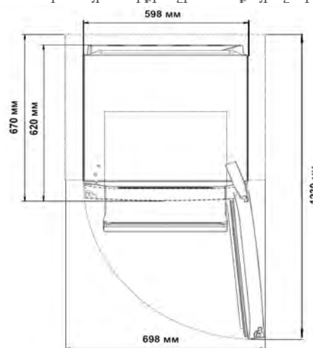
Սառնարանային սարքի աշխատանքային չափերը
