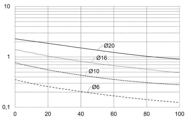
(5) Максимальная скорость: ≤100 (мм/с) Смещение L1: 100 мм
