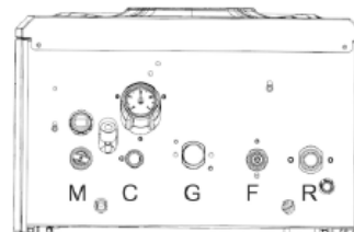
Вид снизу
