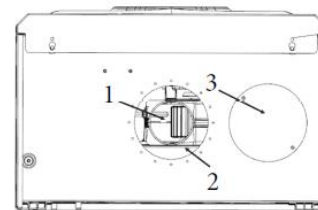
Вид сверху
