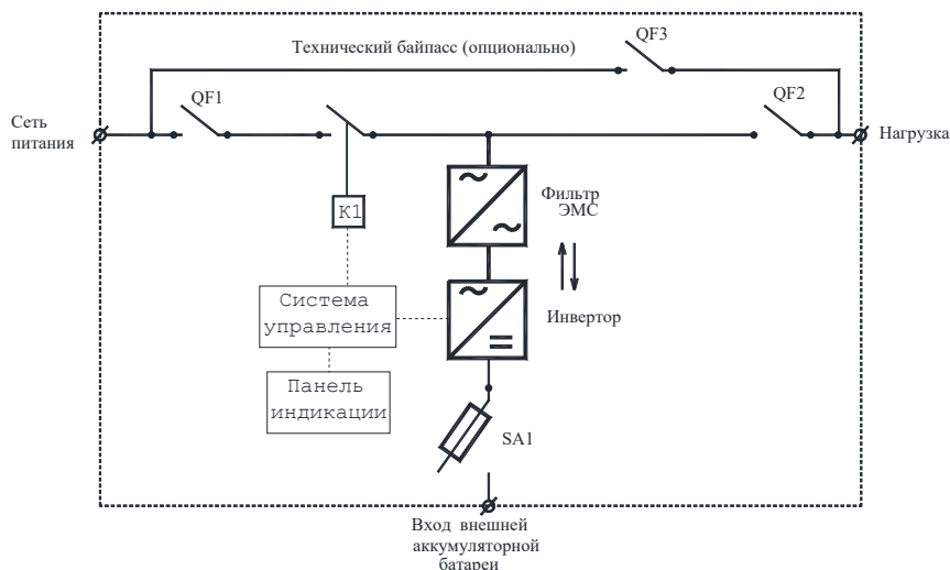
Рис. 3 Структурная схема ИБП
