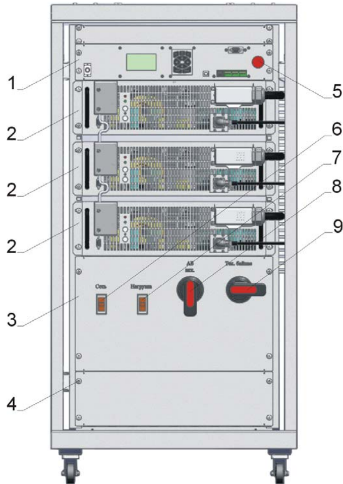
Рис. 1 ИБП РПД-3/3-60-380. Вид спереди.
