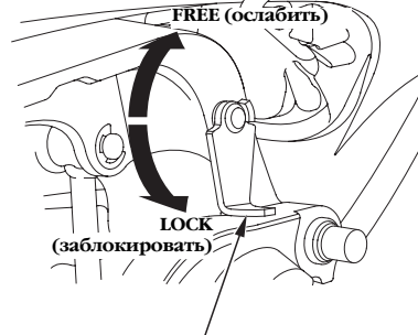
РЫЧАГ ФИКСАТОРА ПОДВЕСНОГО МОТОРА В ПОДНЯТОМ ПОЛОЖЕНИИ
