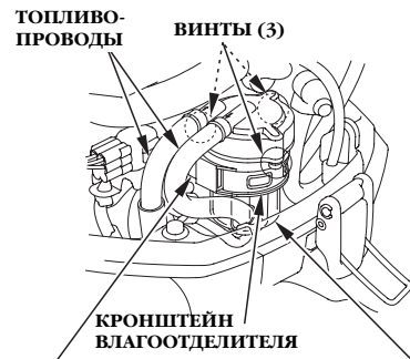
ЛЕНТОЧНЫЙ ХОМУТ ВЛАГООТДЕЛИТЕЛЬ
