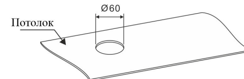
Размер врезного отверстия в потолке - D60мм
