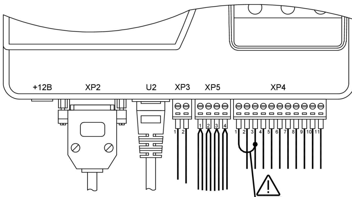
Рисунок 12 – Подключение аккумуляторной батареи лифтового блока
