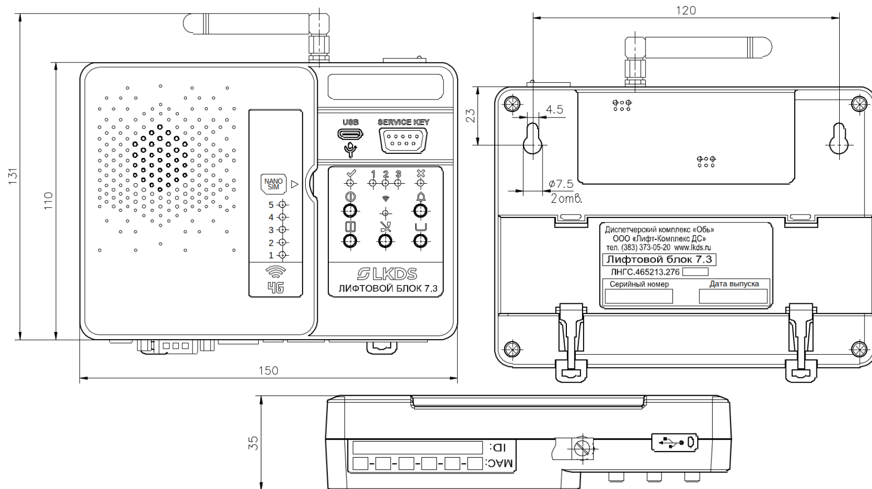
Рисунок А.1 – Габаритные размеры ЛБ7.3
