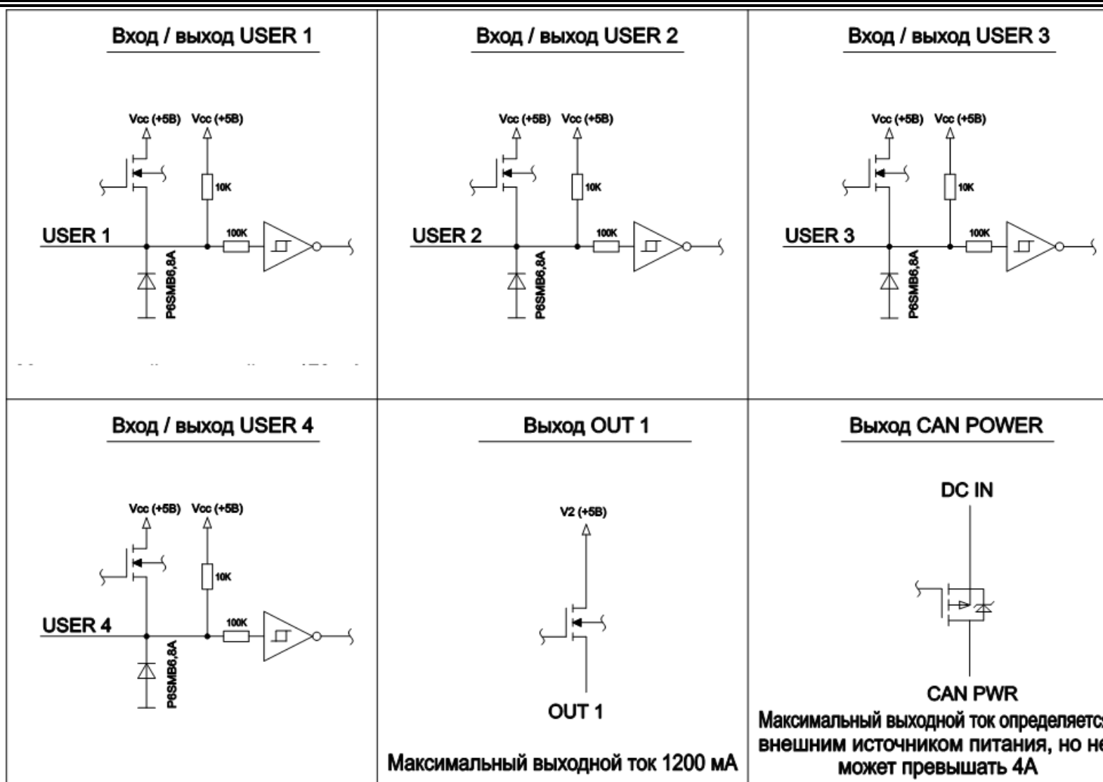
Рисунок Г.1 – Типы входов/выходов лифтового блока 7.3 и варианты их использования
