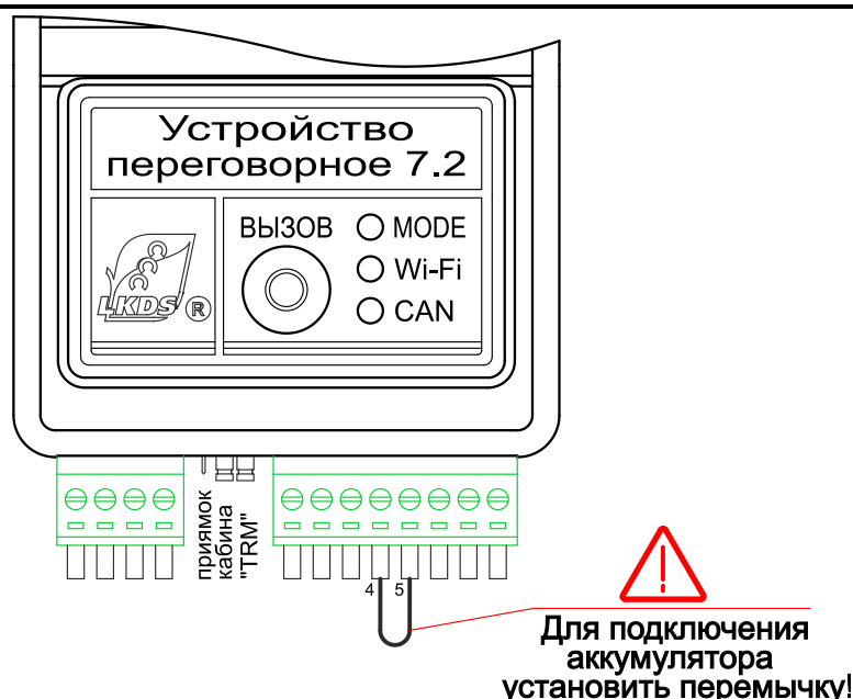
Рисунок 13 – Подключение аккумуляторной батареи переговорного устройства и установка джамперов «Кабина/Приемок»
