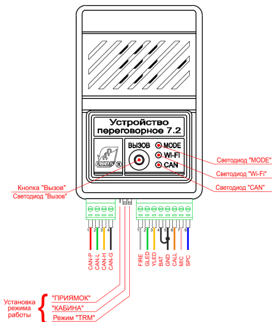
Рисунок 4 – Внешний вид переговорного устройства, назначение разъемов, органов управления и индикации
