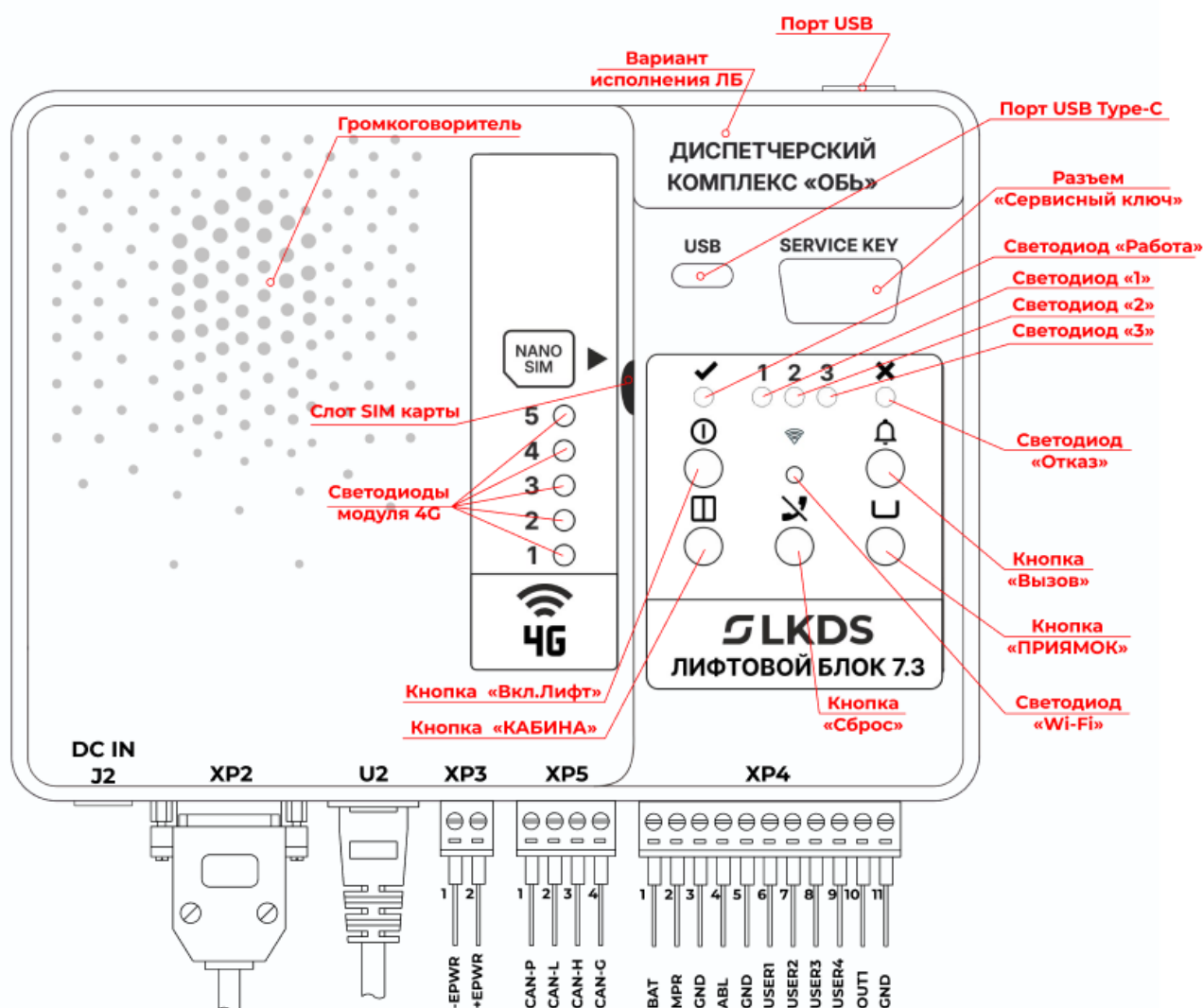
Рисунок 1 – Внешний вид лифтового блока 7.3, назначение разъемов, органов управления и индикации
