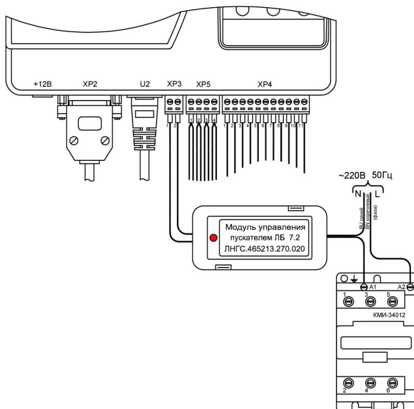
Рисунок 11 – Подключение модуля управления пускателем
