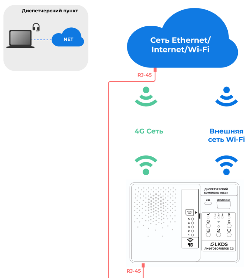
Рисунок 5 – Подключение лифтового блока 7.3 к внешней сети передачи данных
