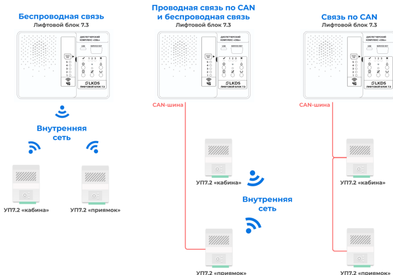
Рисунок 6 – Организация внутренней связи лифтового блока для подключения переговорных устройств 7.2
