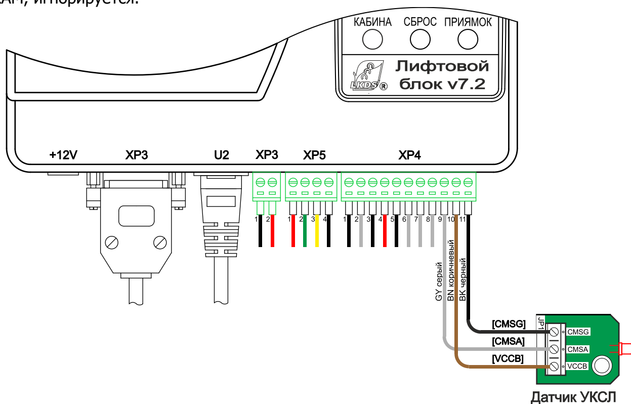
Рисунок 10 – Подключение датчика УКСЛ
