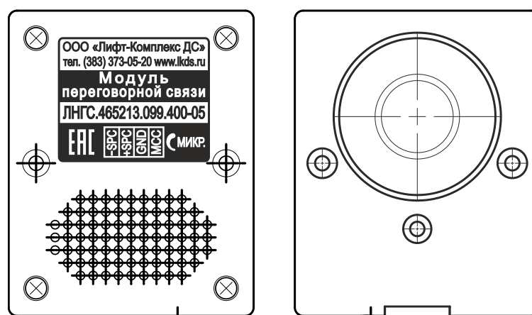
Рисунок 8 – Внешний вид модуля переговорной связи
