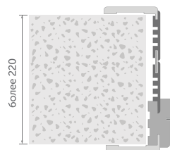
Стыковка с помощью шпонки
