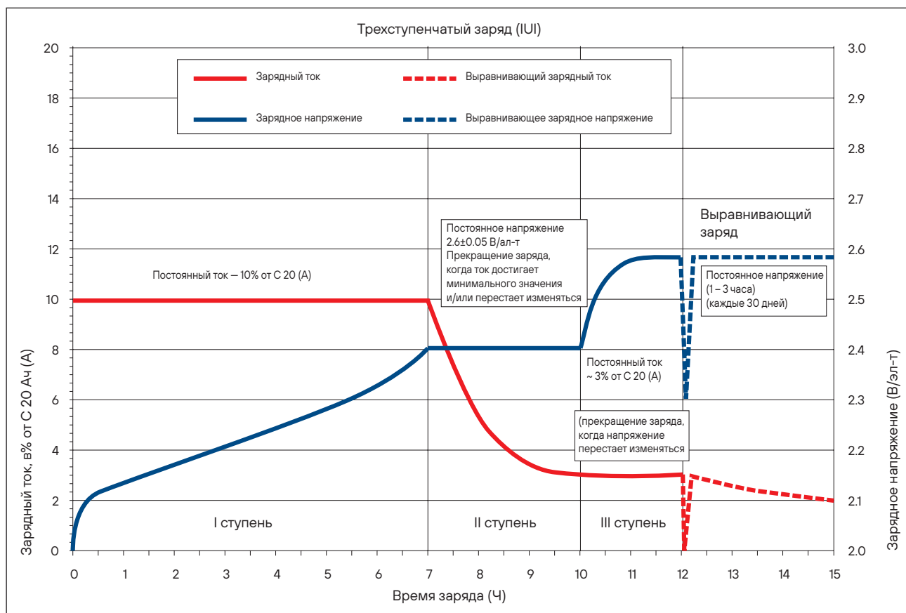
Схема 2: Рекомендуемый график заряда аккумуляторных батарей с жидким электролитом IUI
