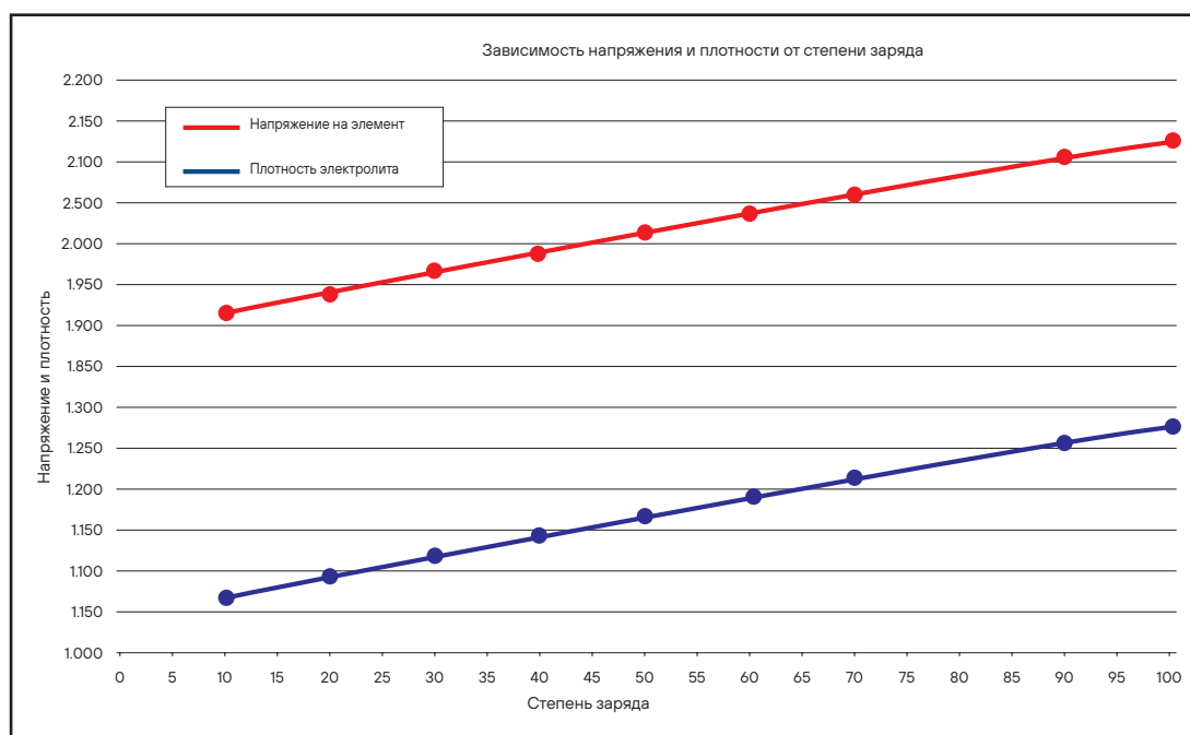
Схема 8: Состояние заряда свинцово-кислотного аккумулятора с жидким электролитом в зависимости от плотности электролита и напряжения холостого хода
