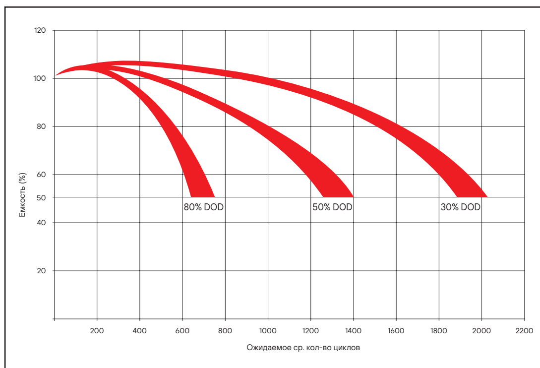
Схема 6: Циклический ресурс в зависимости от глубины разряда.
