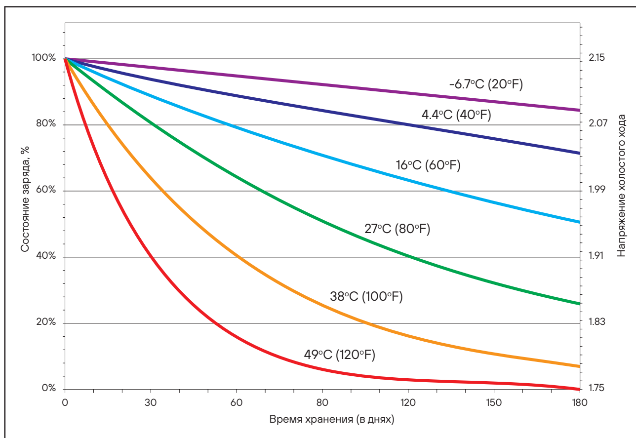
Схема 4: Саморазряд свинцово-кислотного аккумулятора при температуре от -7^{\circ}\text{C} до 49^{\circ}\text{C}
