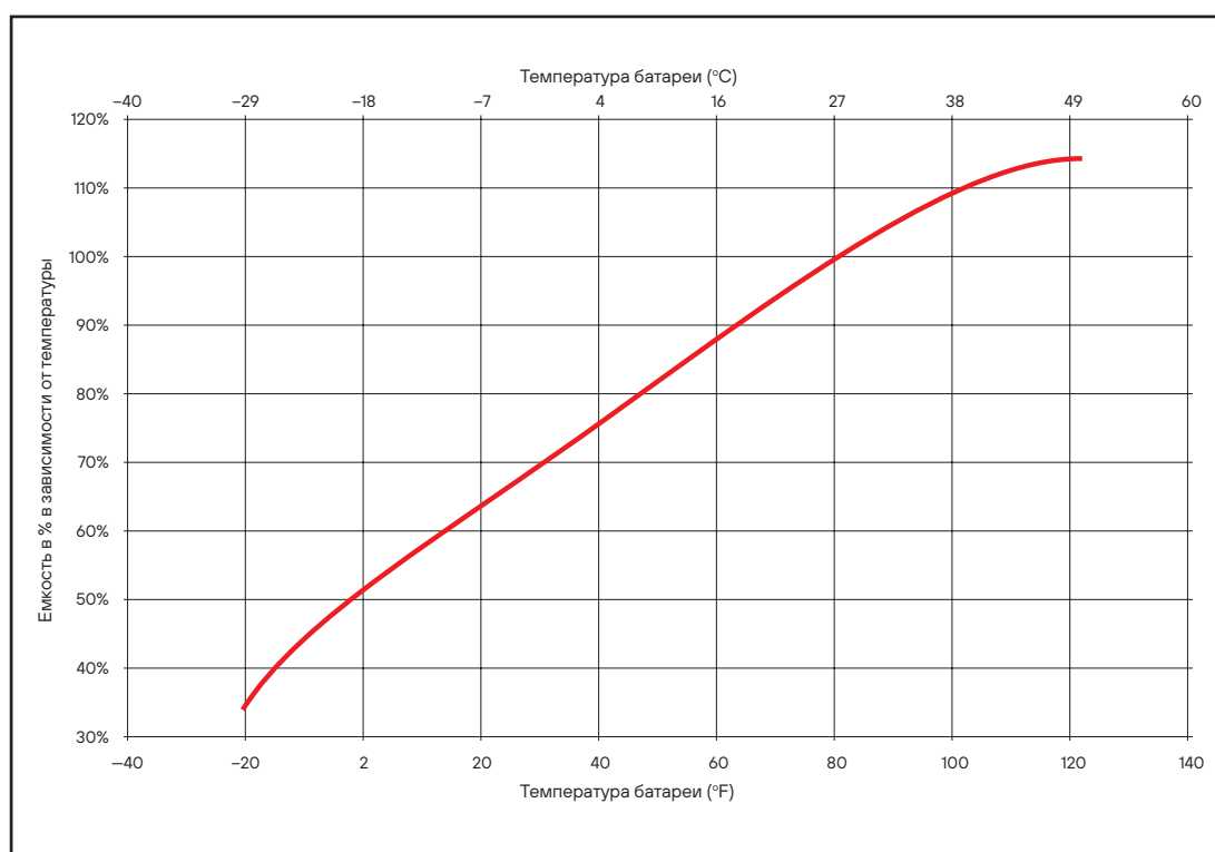
Схема 7: Емкость аккумулятора в % в зависимости от температуры
