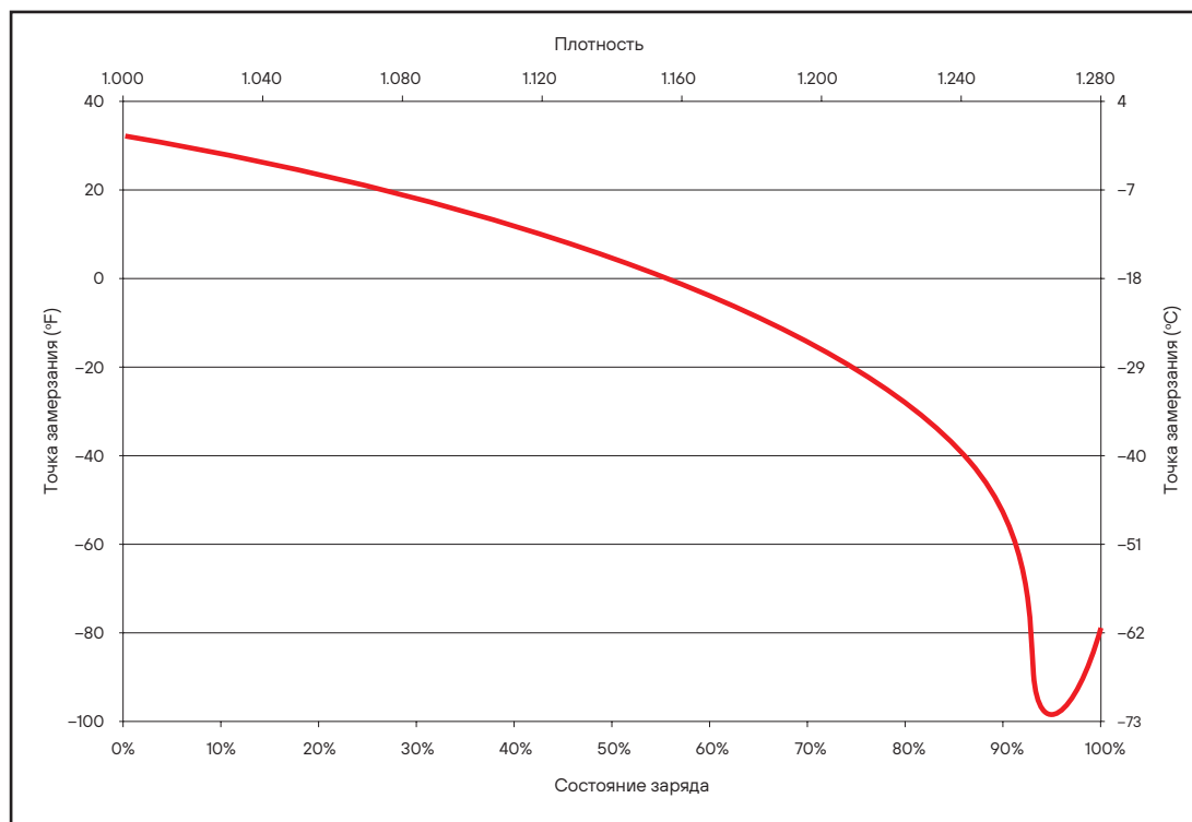
Схема 5: Температура замерзания электролита в зависимости от состояния заряда
