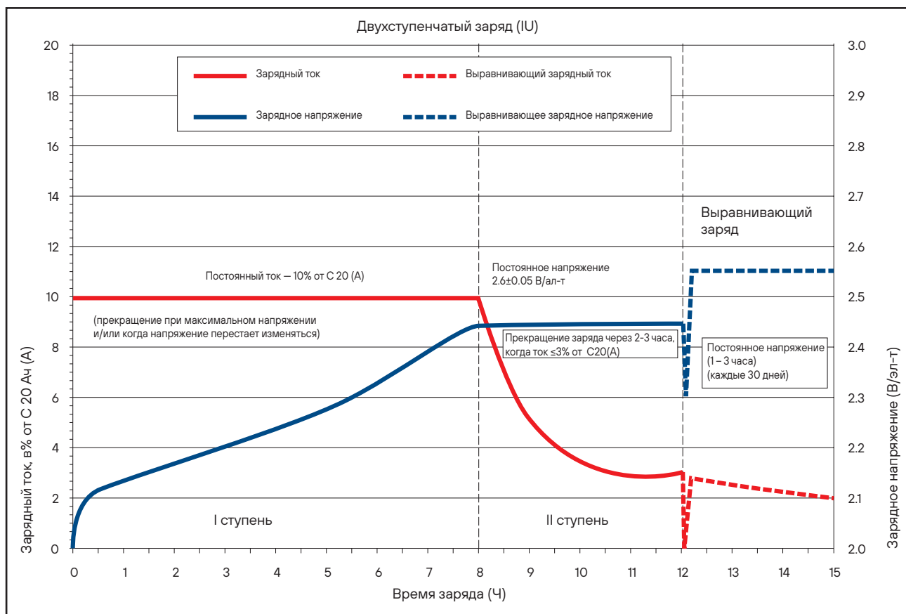
Схема 3: Рекомендуемый график заряда аккумуляторных батарей с жидким электролитом IU
