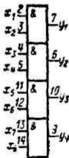
Условное графическое обозначение К172ЛИ1
