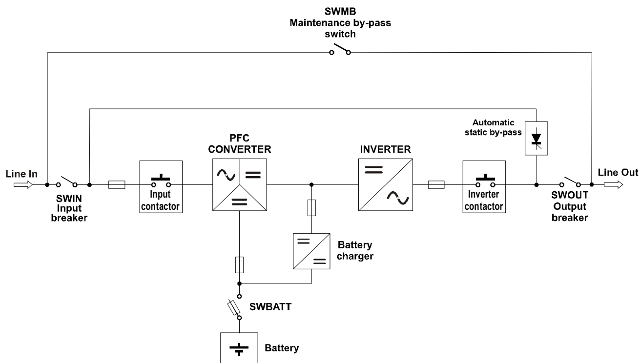
Блок-схема ИБП
