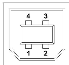
РАЗЪЕМ USB
