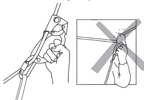
Рис. 6. Нагрузка веревки под углом с щелкиванием карабина в нижнее присоединительное отверстие
