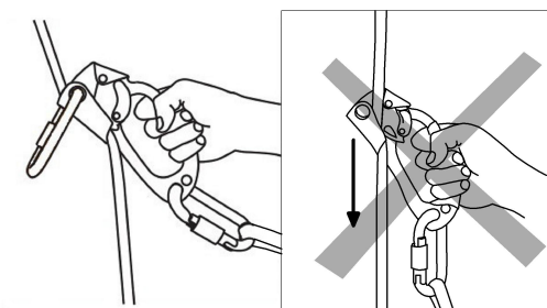
Рис. 7. Нагрузка веревки под углом с щелкиванием карабина в верхнее присоединительное отверстие
