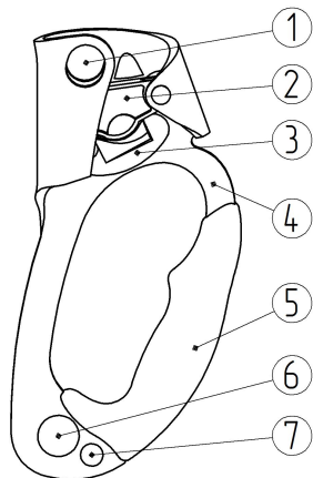
Рис. 1. Зажим ручной «Жумар» правый ver 0101 («Жумар» левый ver 0101-1 является зеркальным отражением):
