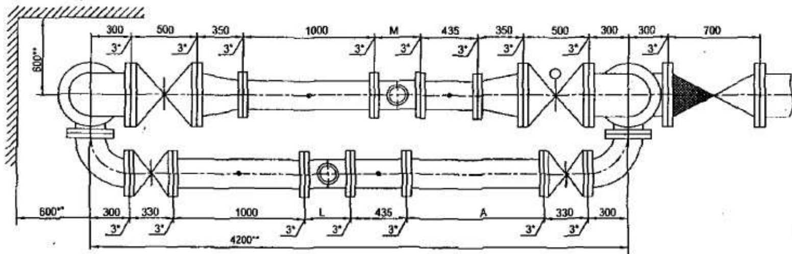
Установка счетчика d_u=200 мм на хозяйственно-питьевой линии и счетчика d_u=200 мм на пожарно-резервной линии в водомерном узле на вводе диаметром 300 мм. Схема водомерного узла.
