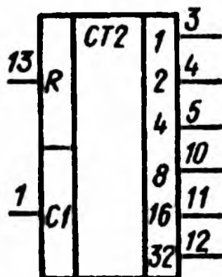
Условное графическое обозначение К176ИЕ1
