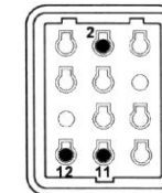
Расположение контактов в интерфейсных разъемах ЭБУ Рис. 2
