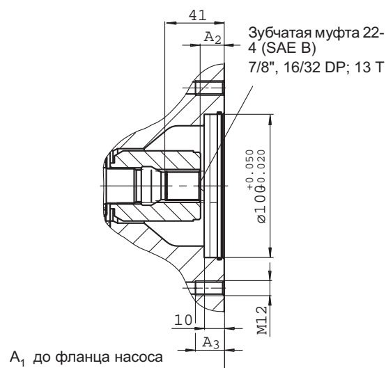
Разрез А - В
