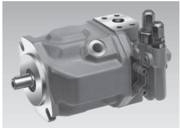
A10VSO...DR
