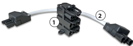
IR-Steckmodul ① mit Adapterkabel ② - 94.2046 IR-Steckmodul ① ohne Adapterkabel - 94.4960
