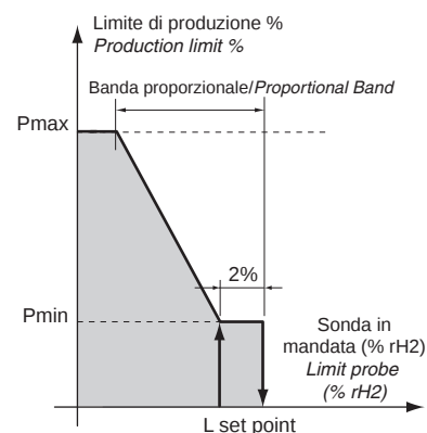
Рис. 14.с Управление датчиком-ограничителем
