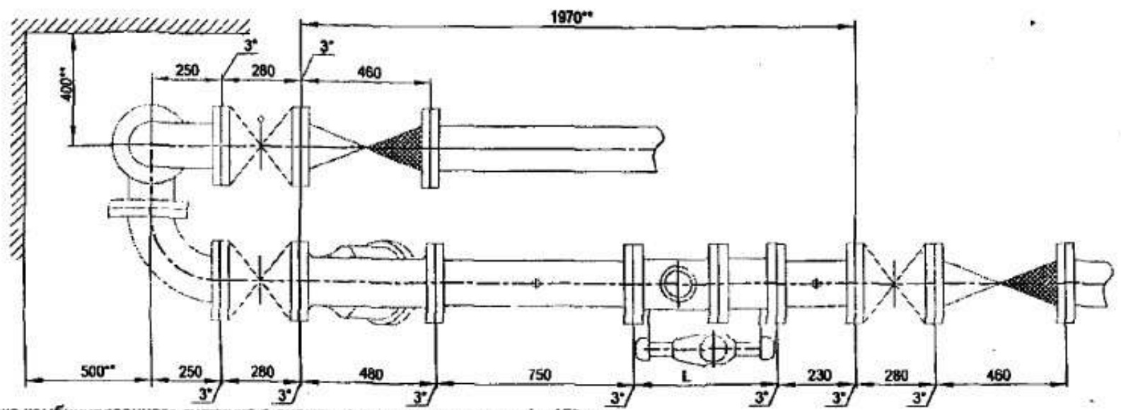
Установка комбинированного счетчика с диаметром основного канала d_u=150 мм с раздельной системой хозяйственно-питьевого и противопожарного водопроводов на вводе диаметром 150 мм.
