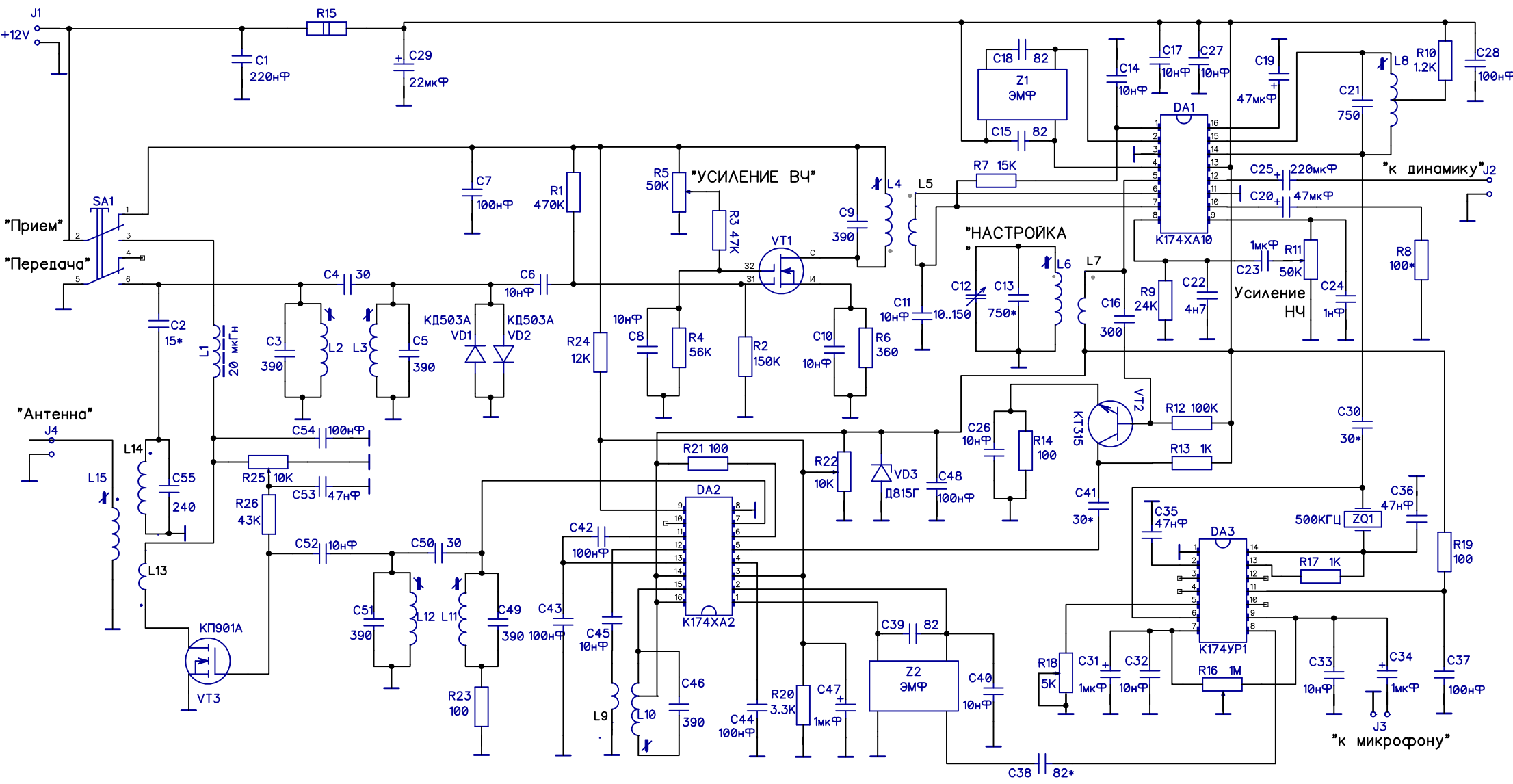
Принципиальная схема Микротрансивера на ИМС серии K174 (РАДИО, 1989, №6)
