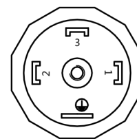
Electrical wiring diagram 电气接线图
