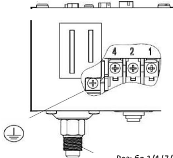
Резьба 1/4 (7/16-20 UNF)
