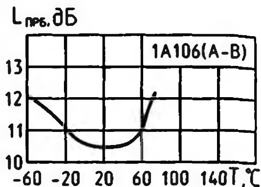
Зависимость потерь преобразования от температуры
