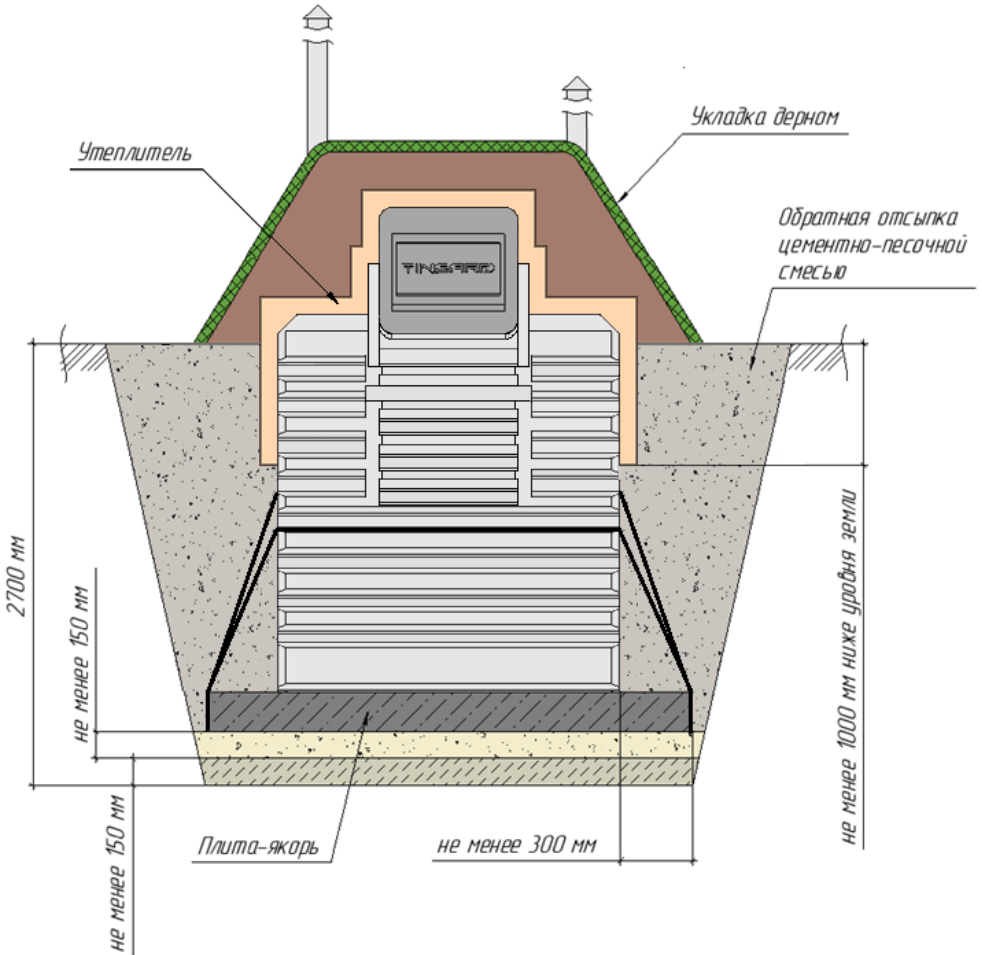
Схема монтажа погреба Т1900БК
