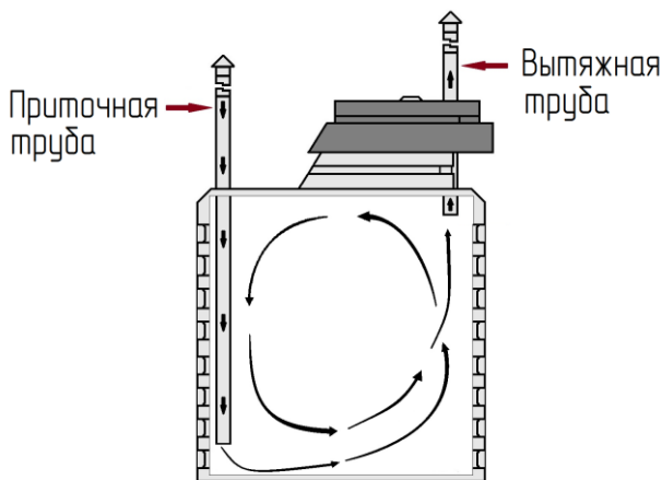
Рисунок 6. Схема циркуляции воздуха в приточно-вытяжной вентиляции.
