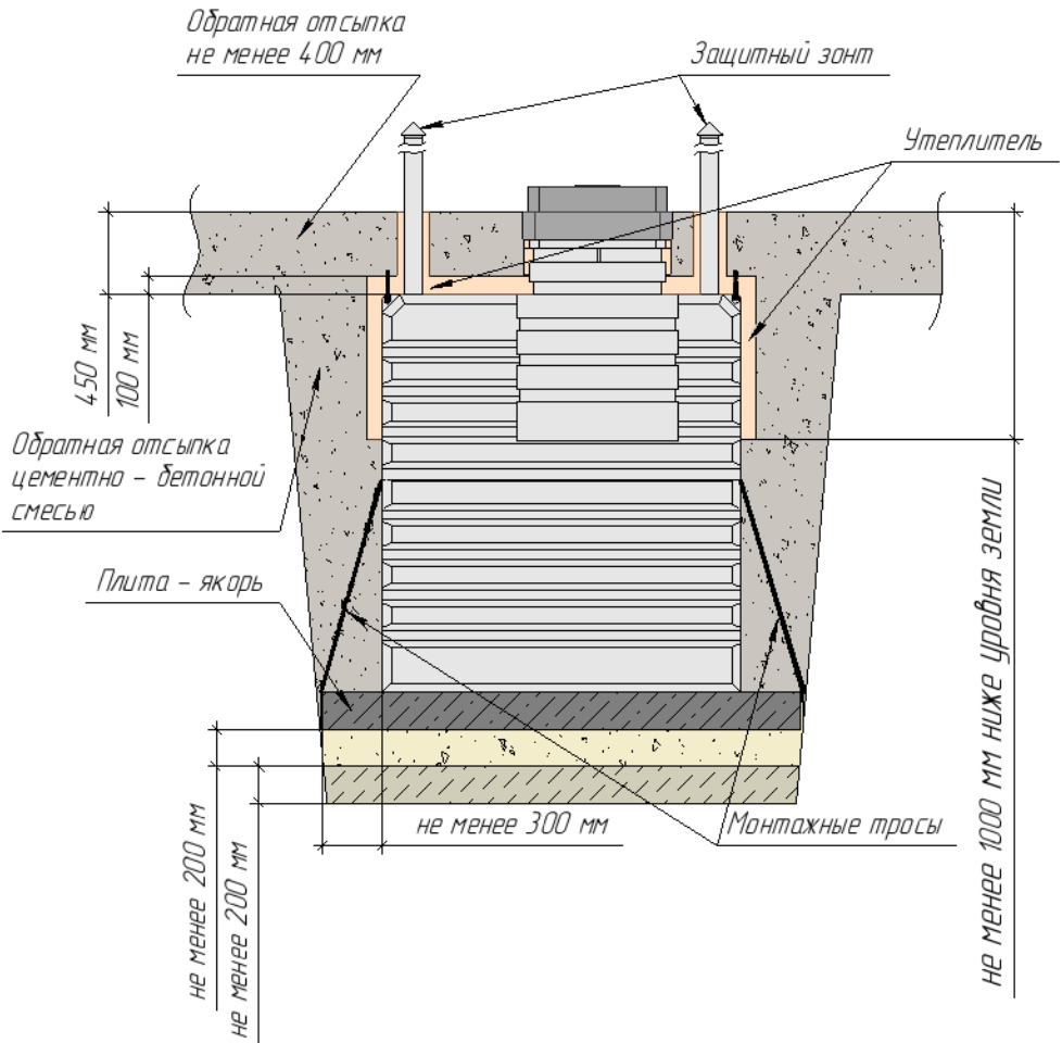
Схема монтажа погреба Т1900К, Т2500К с нижним якорением
