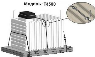
Рисунок 5. Схемы якорения погребов
