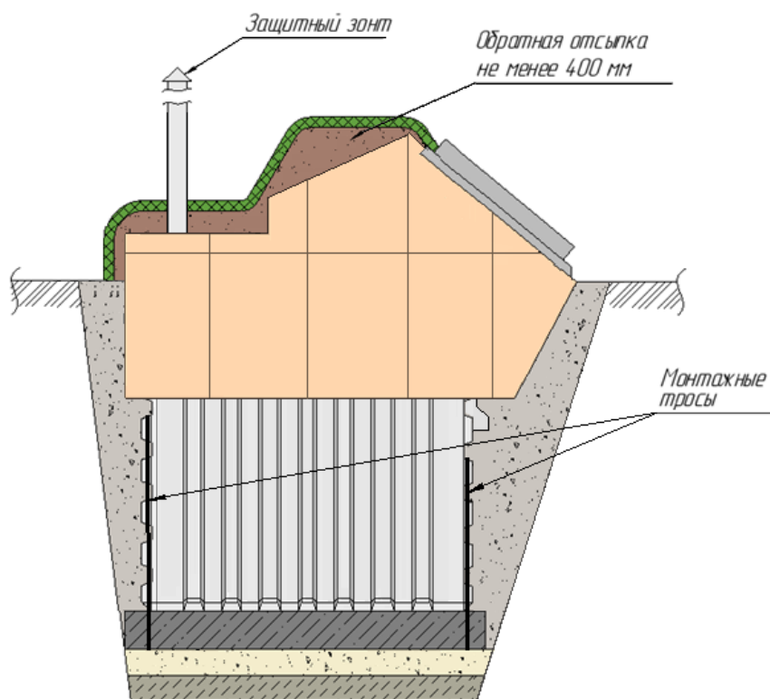
Схема монтажа погребов Т1900БК
