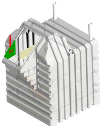
Рисунок 8. Расположение и вид номера на погребе с боковым входом
