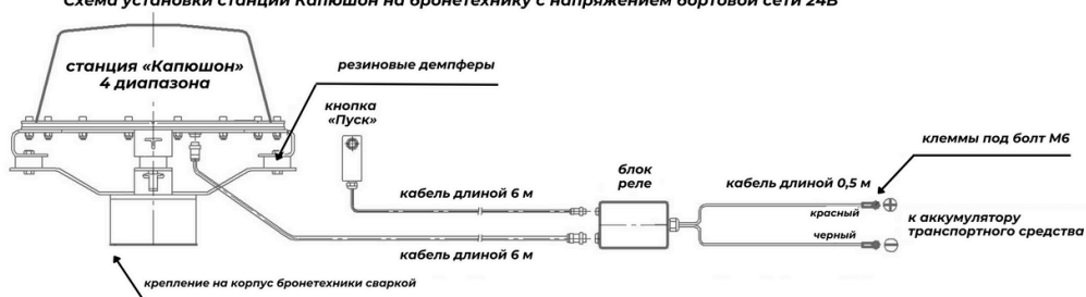
Схема установки станции Капюшон на бронетехнику с напряжением бортовой сети 24В
