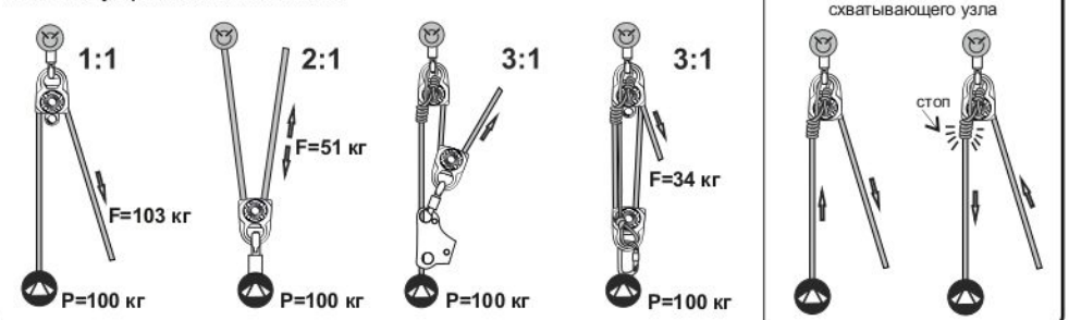
Рис. 4. Популярные схемы полиспастов
