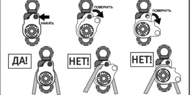
Рис. 6. Раскрытие блок-ролика с вертлюгом
