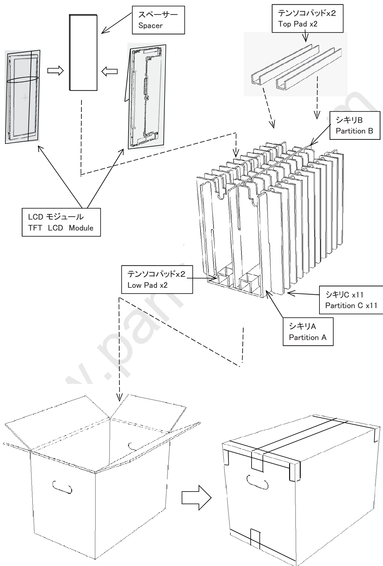
図3: 包装組品図 (Fig3. Packing Form)
