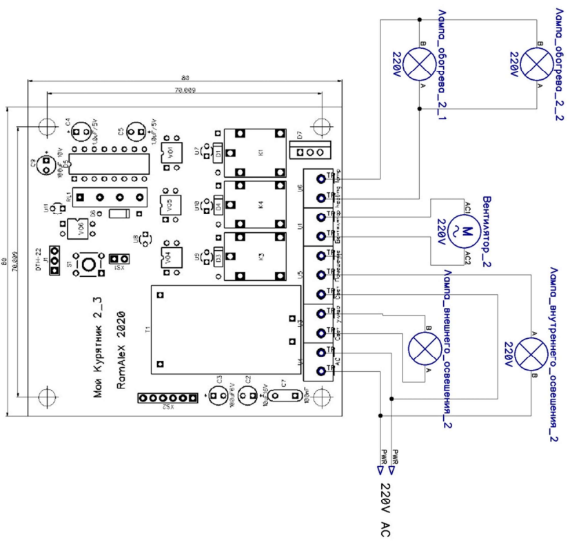
Рис. №2 Схема подключения контроллера (управление освещением в помещении только с приложения)
