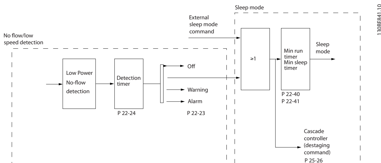
Рисунок 3.16 Обнаружение отсутствия потока
