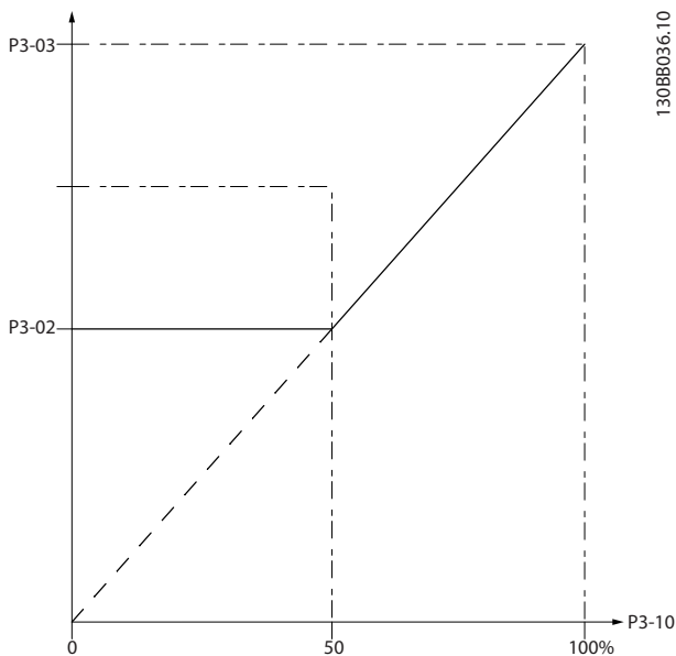
Рисунок 3.4 Задания
