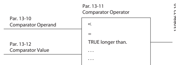
Рисунок 3.14 Компараторы
