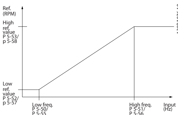
Рисунок 3.9 Импульсный вход
