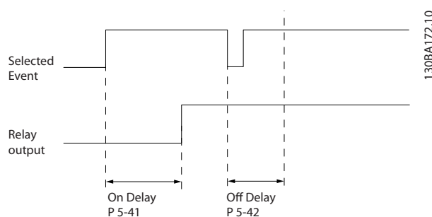
Рисунок 3.8 Задержка выключения, реле
