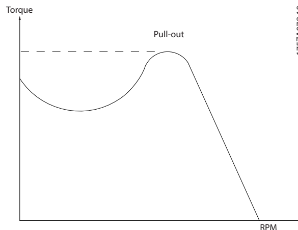
Рисунок 1.1 Момент срыва
