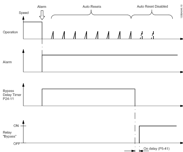
Рисунок 3.18 Функция байпаса
