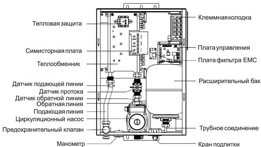
Рис. 1. Конструкция прибора
