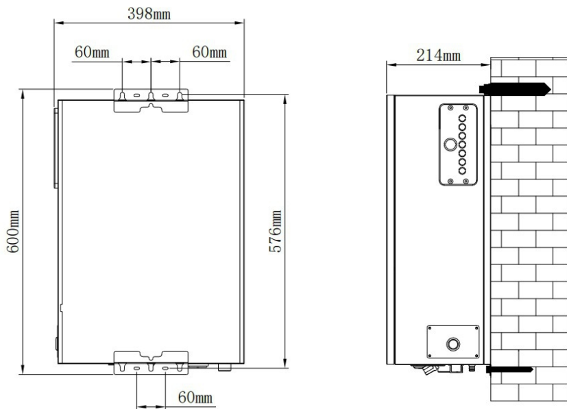
Рис. 4. Размещение прибора
