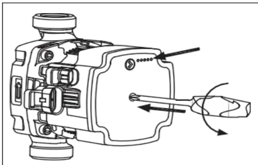
Рис. 8. Обслуживание насоса
