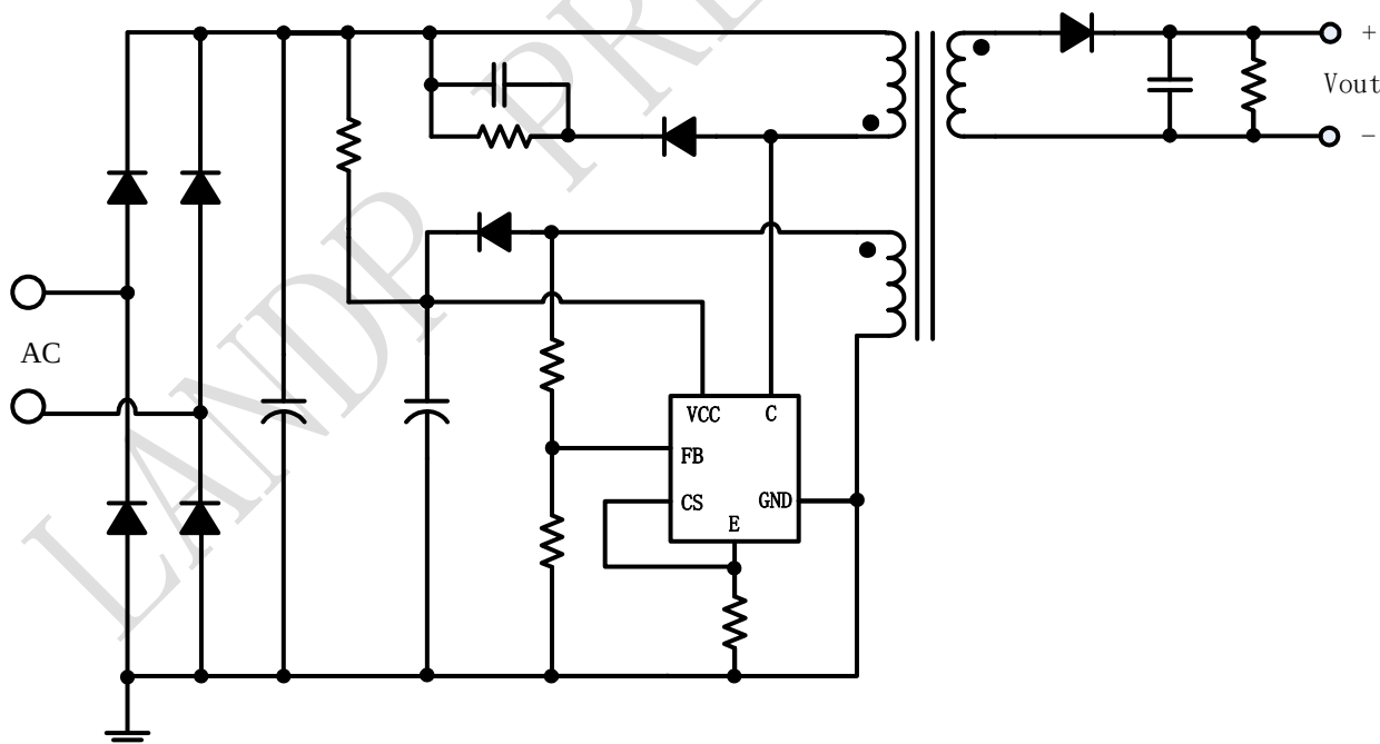
图 1 LP3773D 典型应用图
