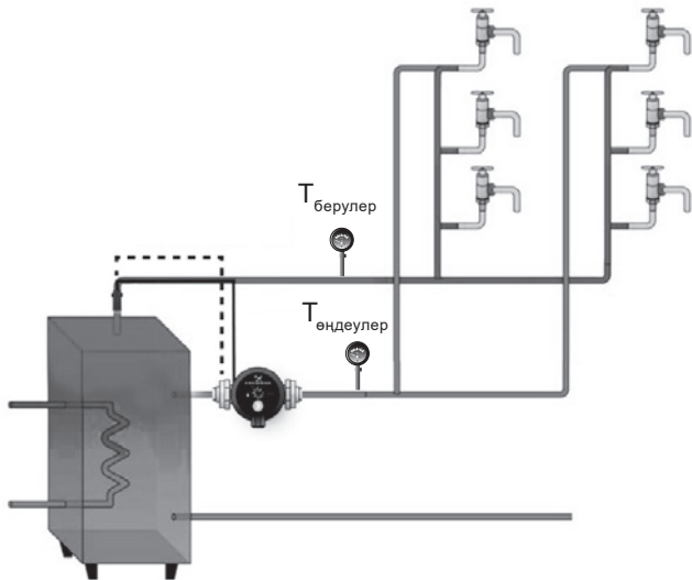
2-сур. Екі температура датчигімен БЖЖ жүйесіндегі COMFORT сорғысы
