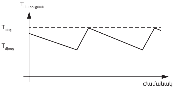
Սկար 3 Ջերմաստիճանի հսկման ռեժիմ
