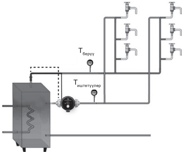
2-сүр. Температуранын эки билдиргичи менен COMFORT соркысмасы ЫСК тутумунда
