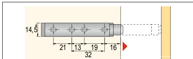
Механизм открывания дверей без ручек
