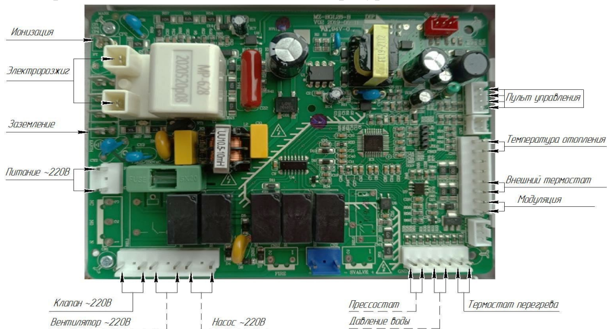
Рисунок 2 - Схема электрических подключений котла AXIS-09-07...25E(W)-00
