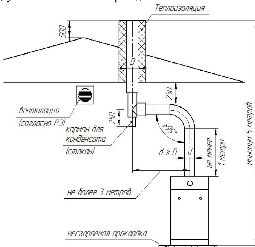
Рисунок 8 – схема монтажа дымохода.
