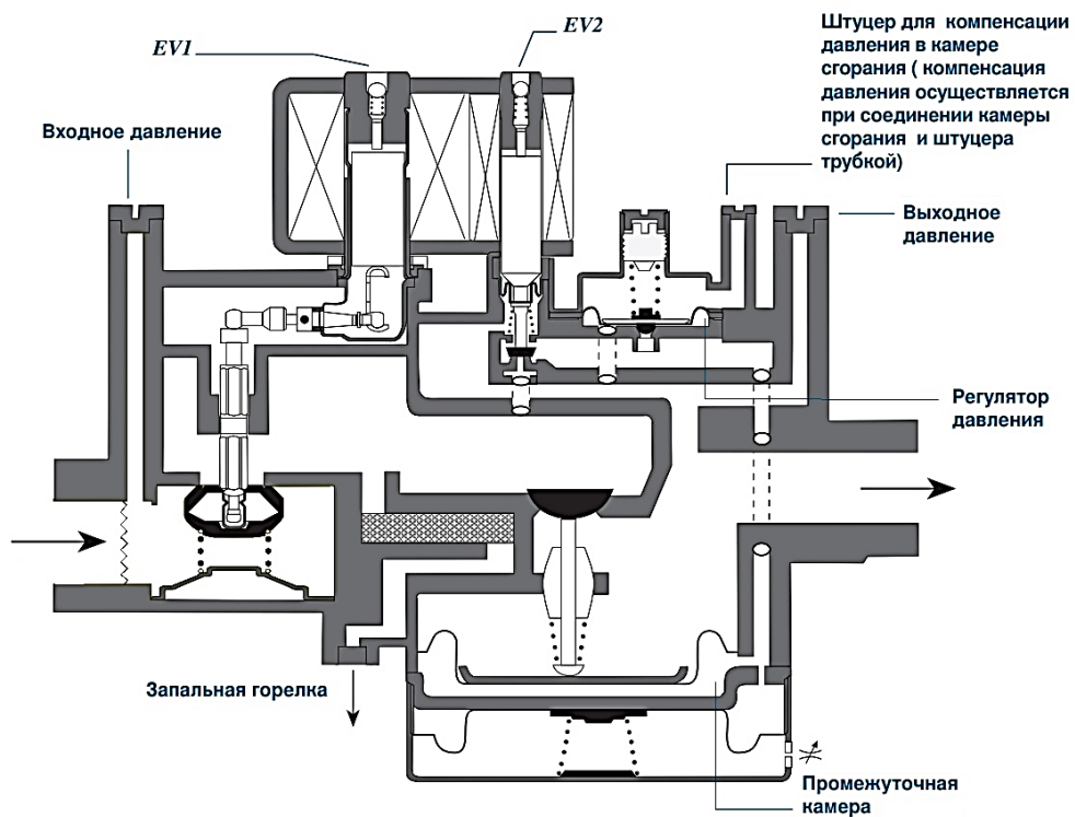
Рисунок 4б – Конструкция клапанов SIT 840 SIGMA и ERCO EBR2006N.
