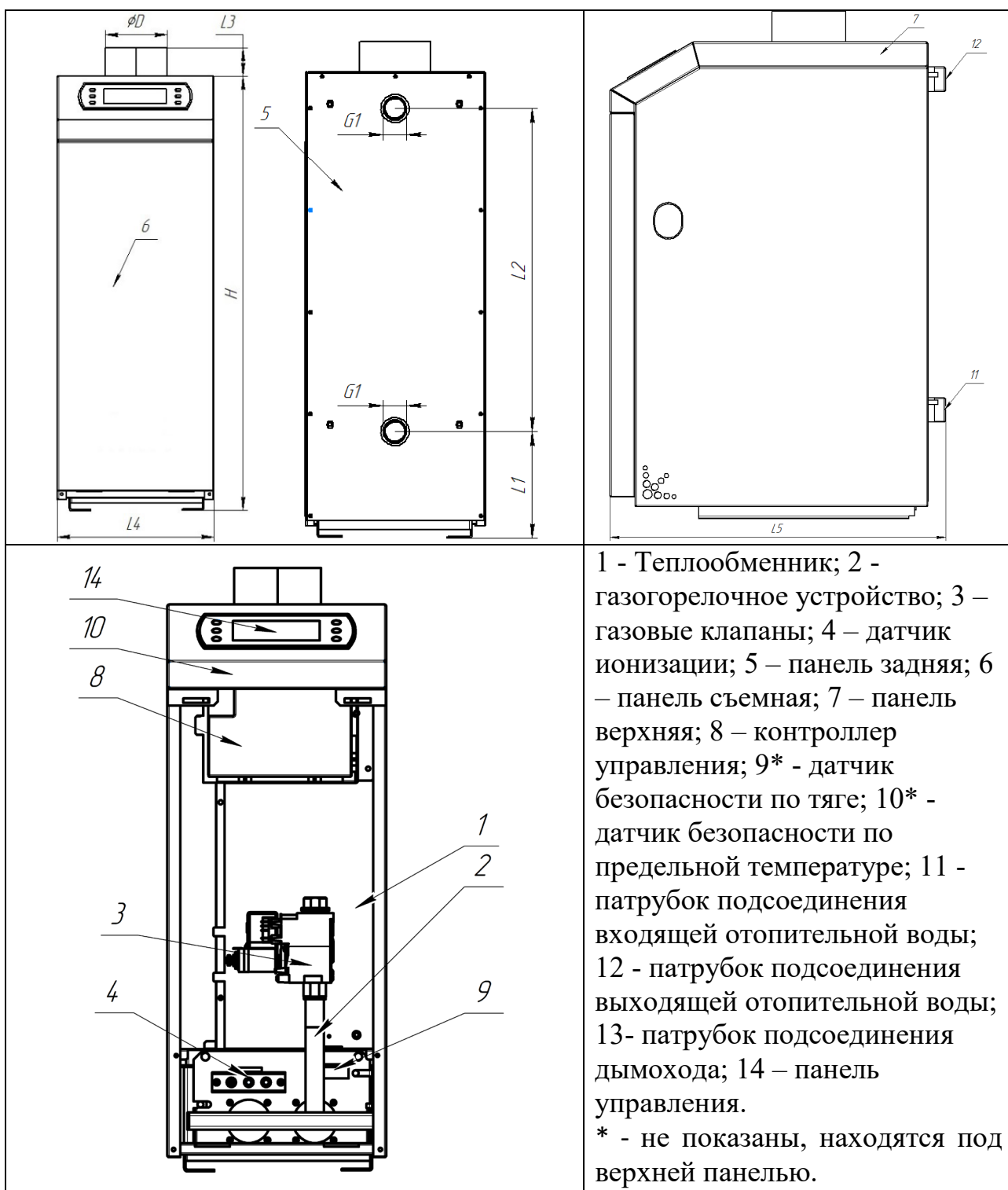
Рисунок 1 – конструкция котла AXIS SMART
