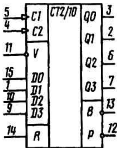
Условное графическое обозначение К555ИЕ6
